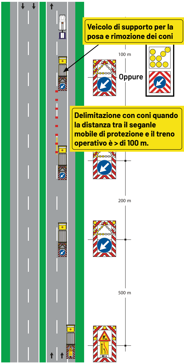
Layout del cantiere rielaborato sulla base della Tavola 41 del Disciplinare Tecnico 2002
