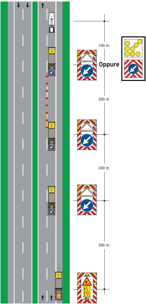
Layout del cantiere rielaborato sulla base della Tavola 41 del Disciplinare Tecnico 2002
