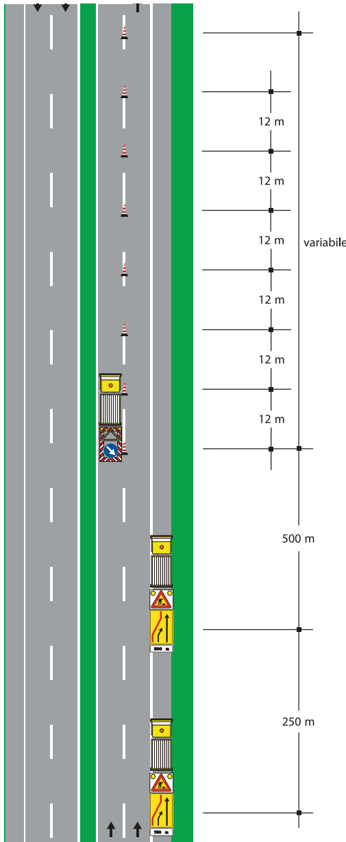
Layout del cantiere rielaborato sulla base della Tavola 40 del Disciplinare Tecnico 2002
